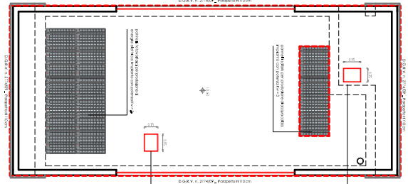
PIANTA COPERTURA
