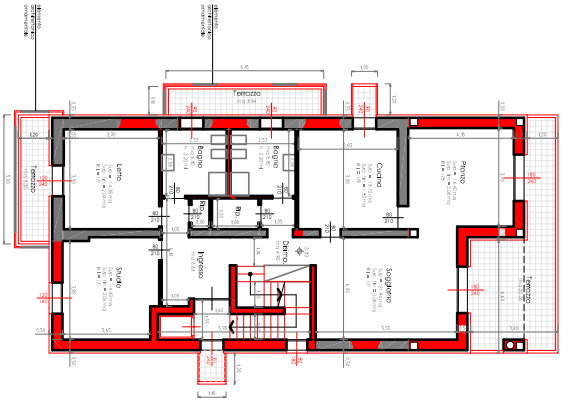
PIANO PRIMO
