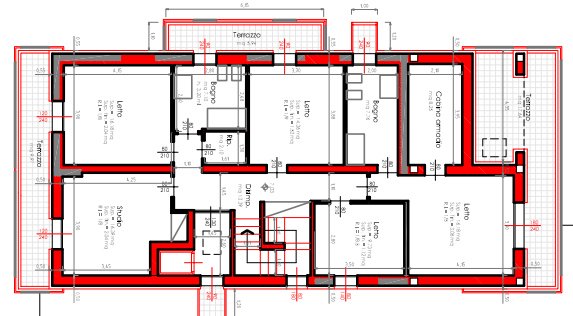
PIANO SECONDO
